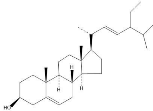
2. Стигмастерол
