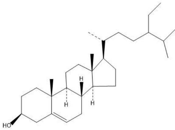
1. Бета-ситостерол
