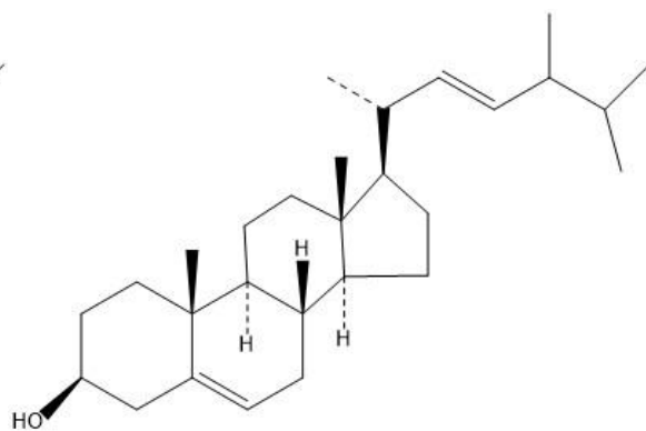
4. Брасикастерол
