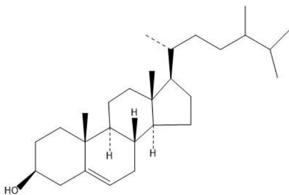
3. Кампестерол
