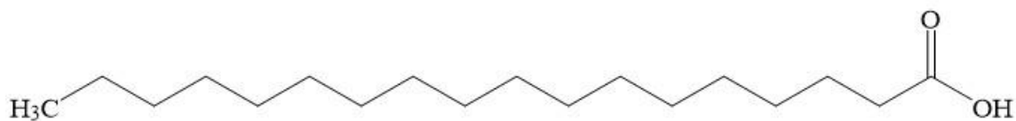
Рисунок 8 - структурная формула стеариновой (октадекановой) кислоты ( C_{18:0} ) Брутто-формула: C_{18}H_{36}O_2
