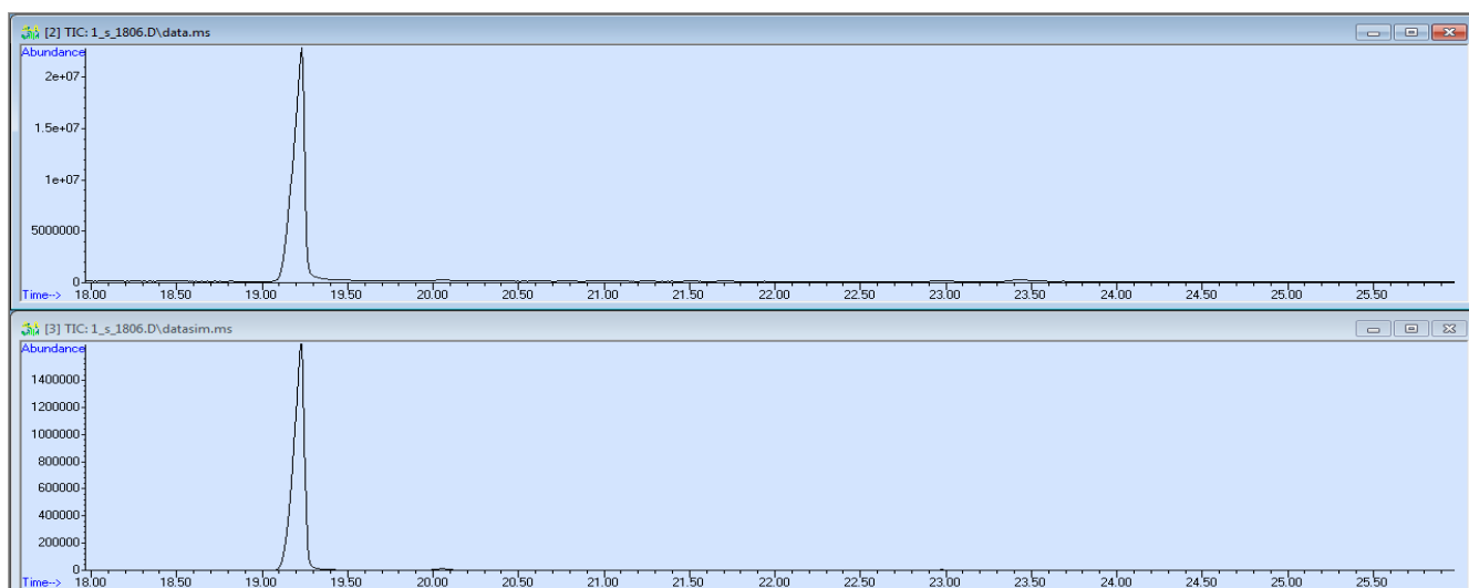
Рисунок 14 - Хроматограмма стероидной фракции молочного жира пробы молока, пик холестерина, характерный для стандартной продукции (код образца 1806).
