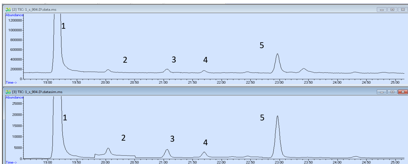
Рисунок 23 - Хроматограмма стериновой фракции молочного жира нестандартной пробы сливочного масла. Основной пик 1 – холестерин; дополнительные пики: 2 – brassикастерин, 3 – кампестерин, 4 – стигмастерин, 5 – бета-ситостерин (код образца 904)
