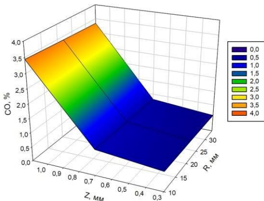
Рис. 1. Зависимость содержания CO, %, от зазора в свече зажигания Z , мм, и эквивалентного сопротивления каталитического нейтрализатора R , мм (при постоянном значении пропускной способности электромагнитной форсунки, равном 106...
